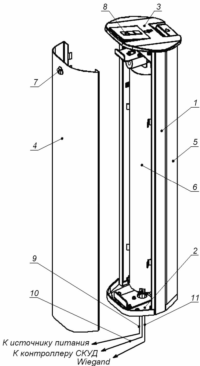
Рисунок 2 Устройство картоприемника
