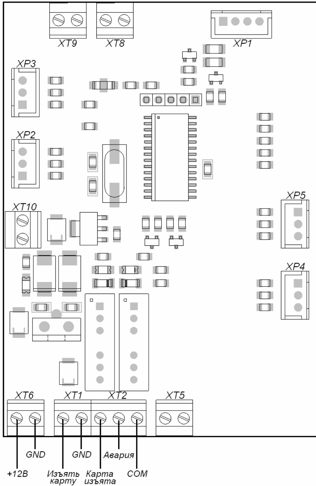
Рисунок 4 Плата управления картоприемником
