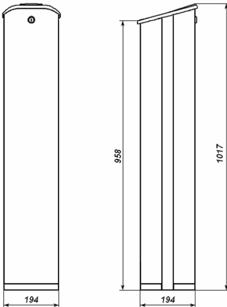
Рисунок 1 Габаритные размеры картоприемника
