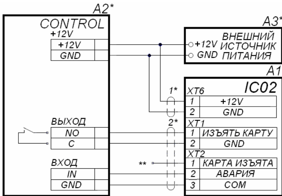
Рисунок 7 Схема подключения картоприемника к контроллеру СКУД
